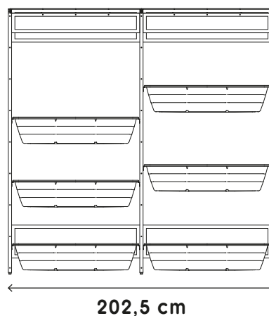
LARGHEZZA FRONTALE
